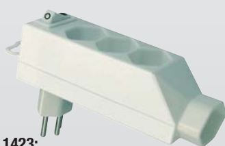
1423: Abzweigstecker T13, drehbar mit Schalter / Fiche de dérivation T13, pivotante avec interrupteur 3x T13 horizontal + 1 x T13 vertikal für permanenten Anschluss / 3x T13 horizontale + 1 x T13 verticale pour le branchement permanent
