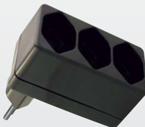
1313: Abzweigstecker T13 Rechteckgehäuse / Fiche de dérivation T13, boîtier rectangulaire 3x L+N+PE
